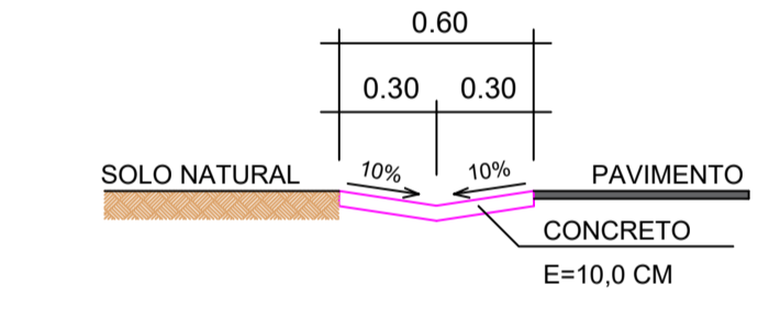
PERFIL ESQUEMÁTICO - SARJETÃO
