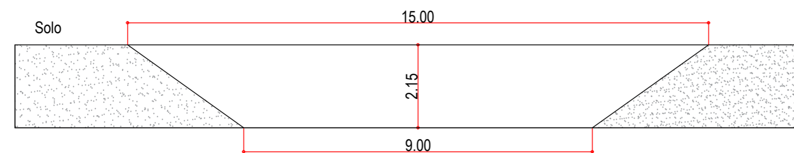
PERFIL NATURAL DO TERRENO ESCALA 1:100
