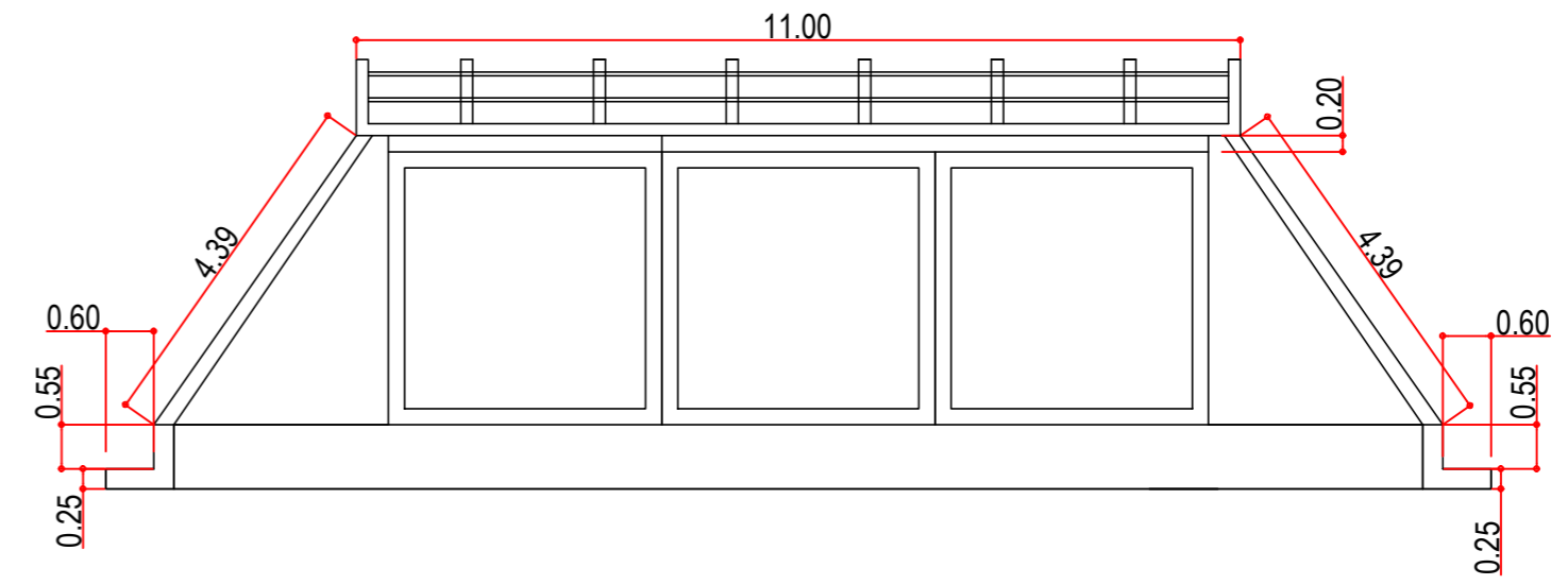
VISTA LONGITUDINAL DA PONTE ESCALA 1:100
