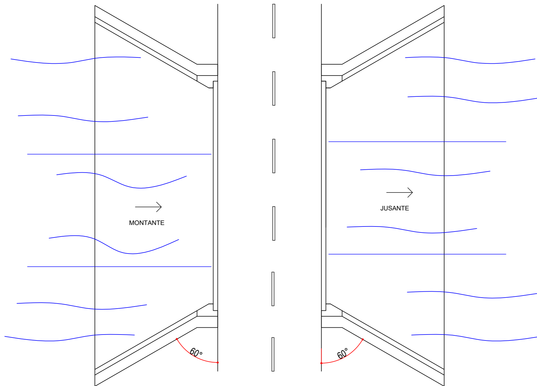
IMPLANTAÇÃO ESCALA 1:100
